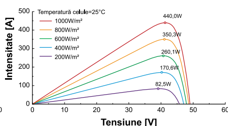
Curba putere - Tensiune
