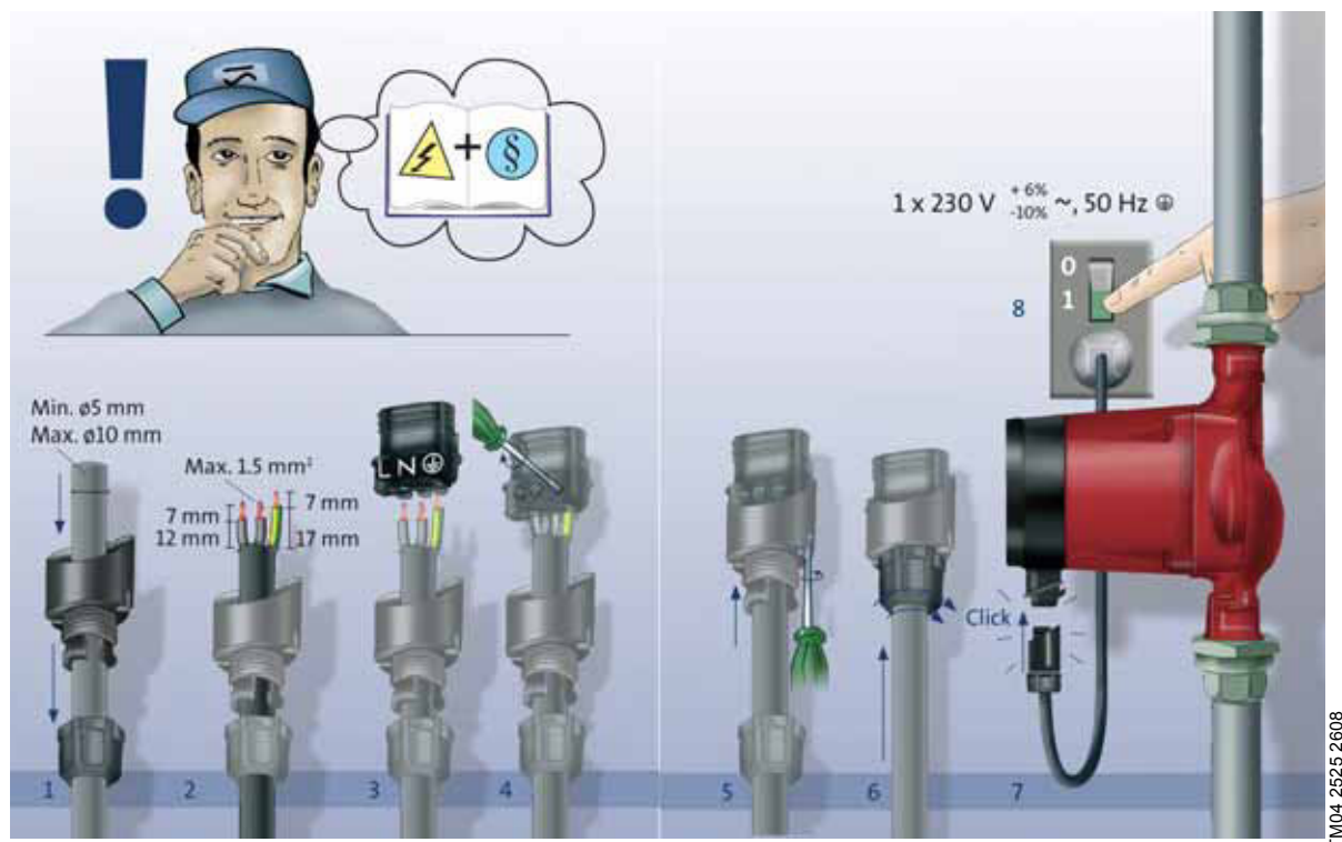
Fig. 6 Conexiunea electrică
