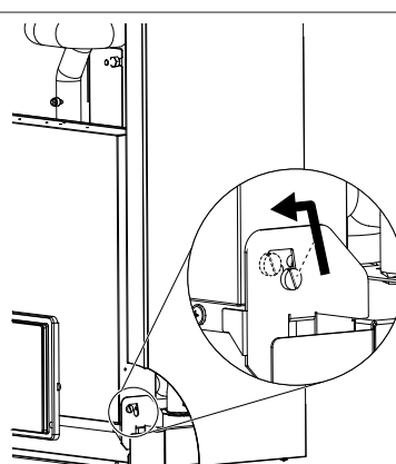
fig. 18 - cum se deblochează caseta electrică
