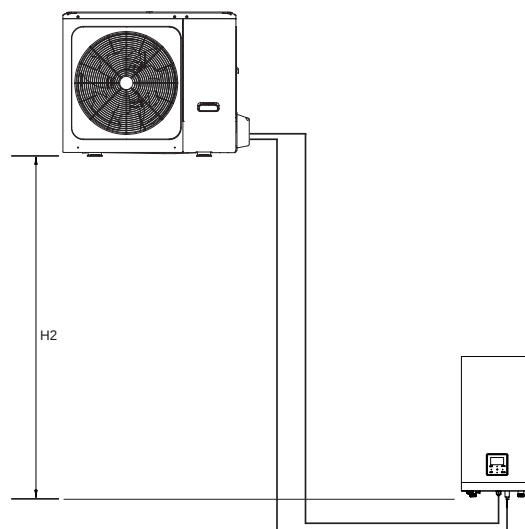
fig. 9 - Unitate extern dedesubtul unității interne
