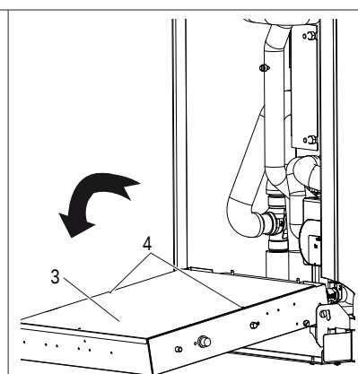
fig. 19 - cum se rotește caseta electrică
