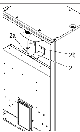
fig. 17 - vedere f r panoul frontal
