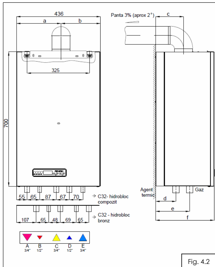
Fig. 4.2 Dimensiuni de gabarit si pozitie de montaj.
