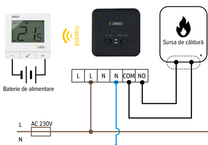
a) Scheme de conectare la sursa de căldură
