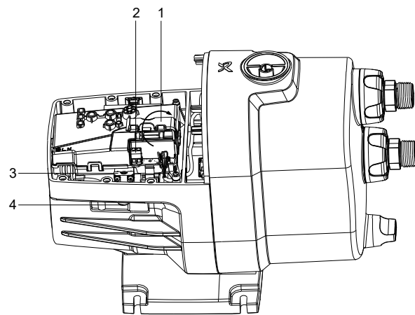
Conectarea intrării externe
