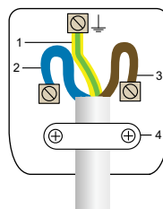
Exemplu, cablare fișă
