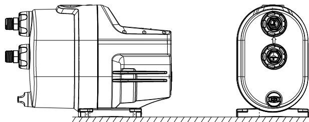
Fundația orizontală
